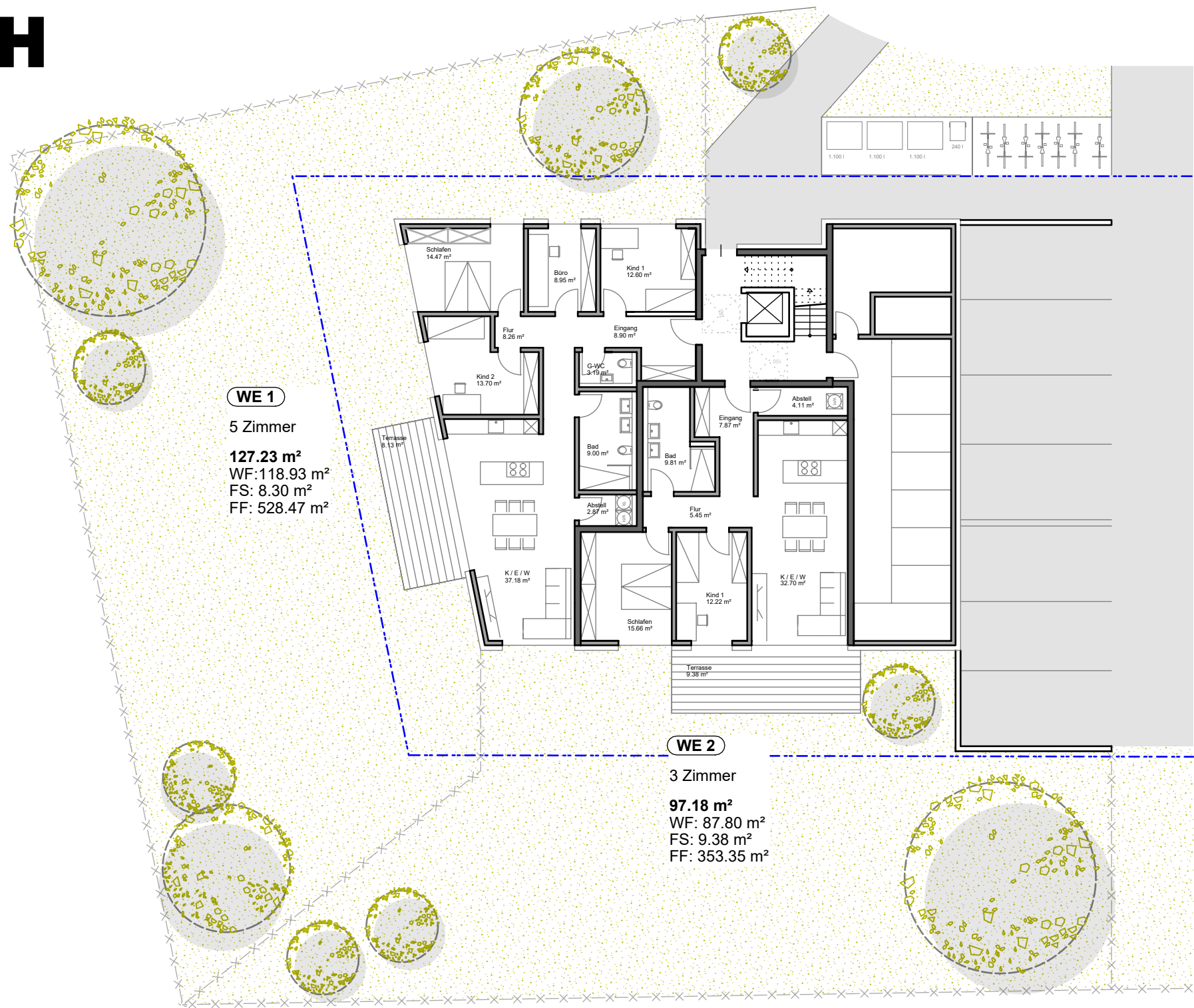
ERDGESCHOSS
