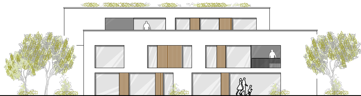
ANSICHT WEST
