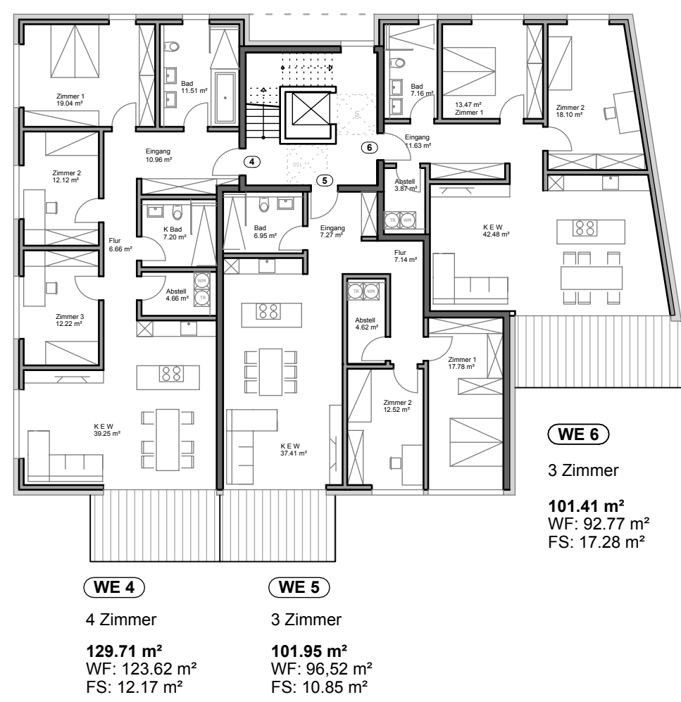
OBERGESCHOSS
