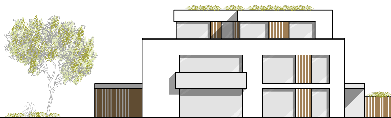
ANSICHT OST
