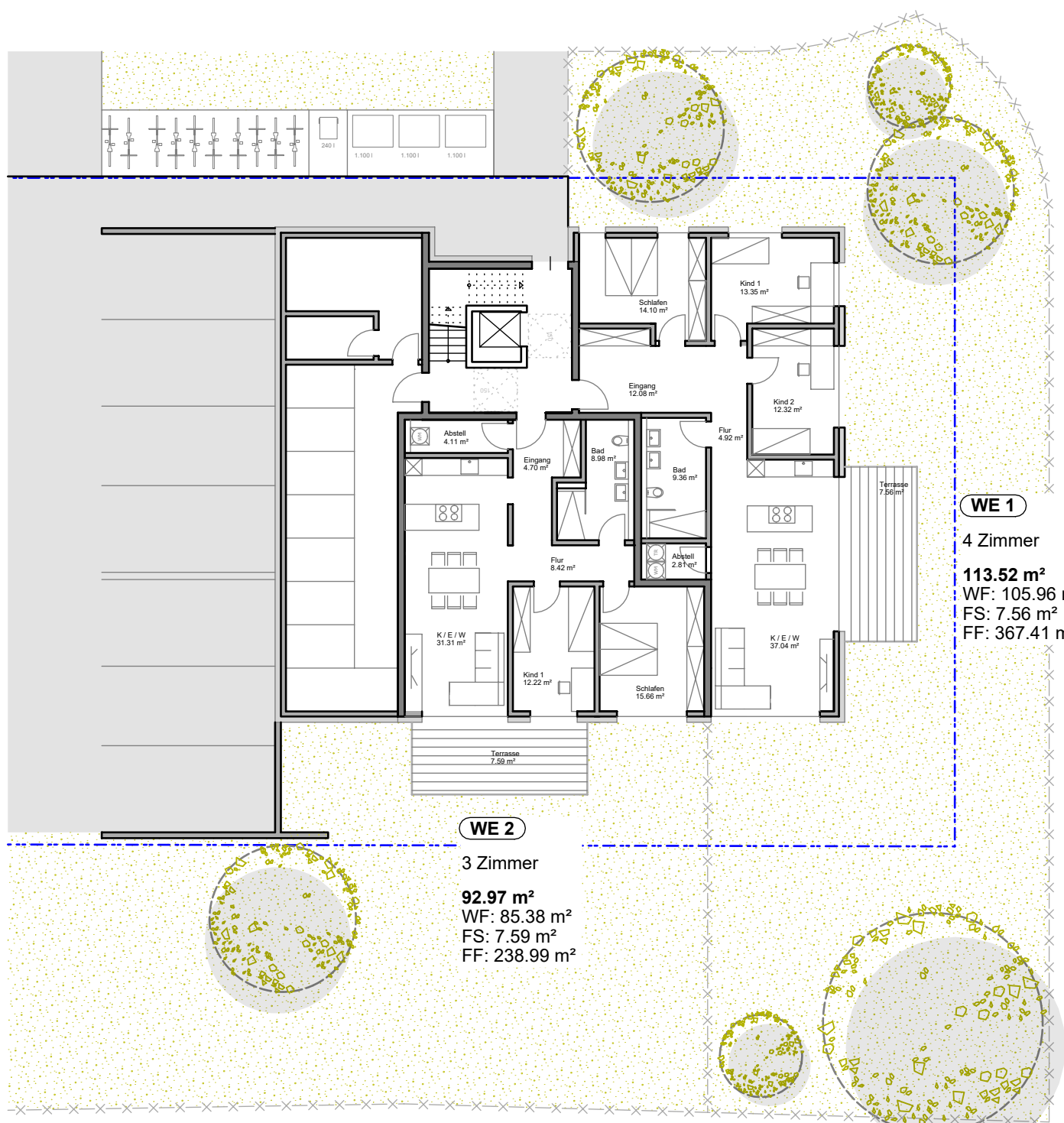
ERDGESCHOSS
