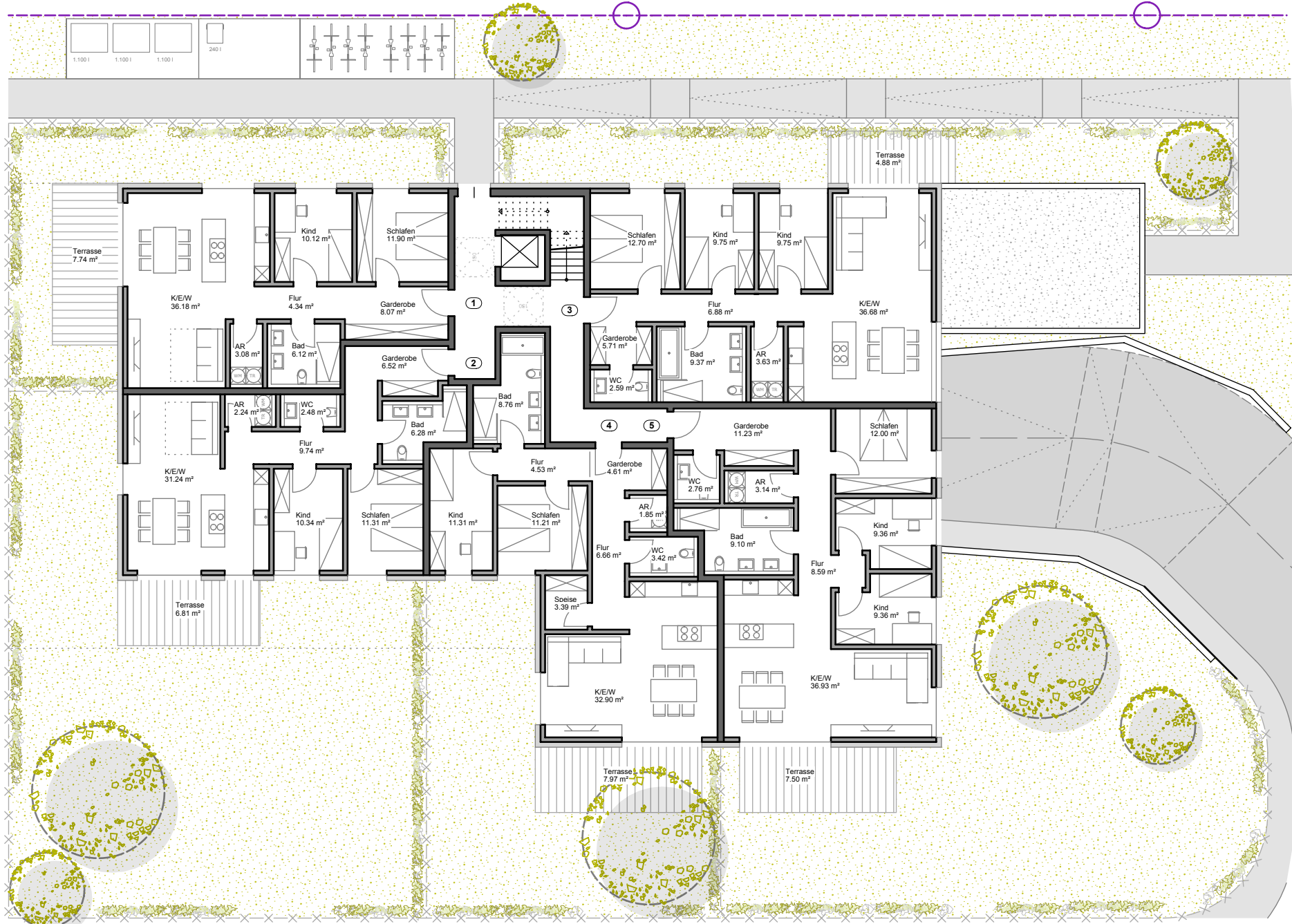
ERDGESCHOSS
