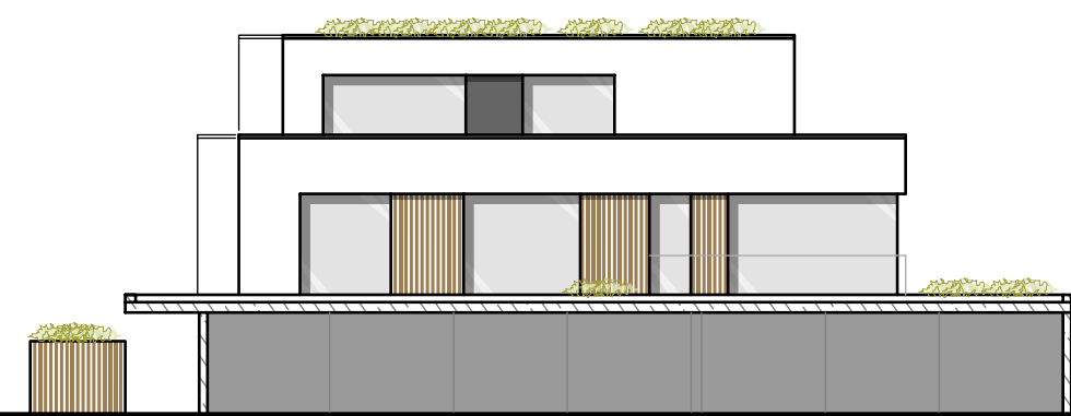
ANSICHT WEST
