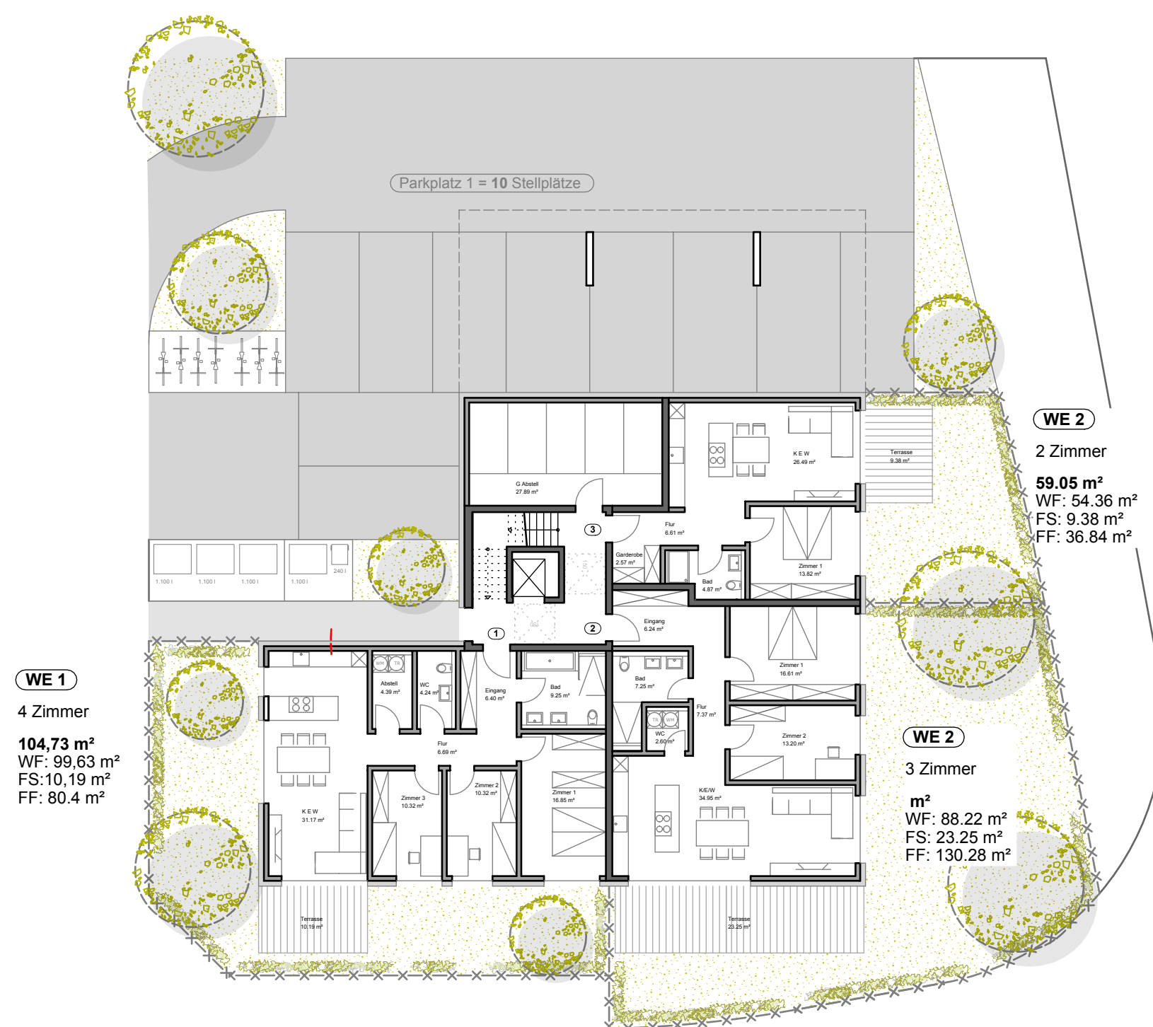
ERDGESCHOSS
