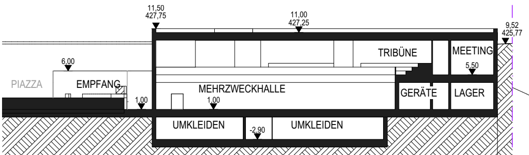
Schnitt Mehrzweckhalle
