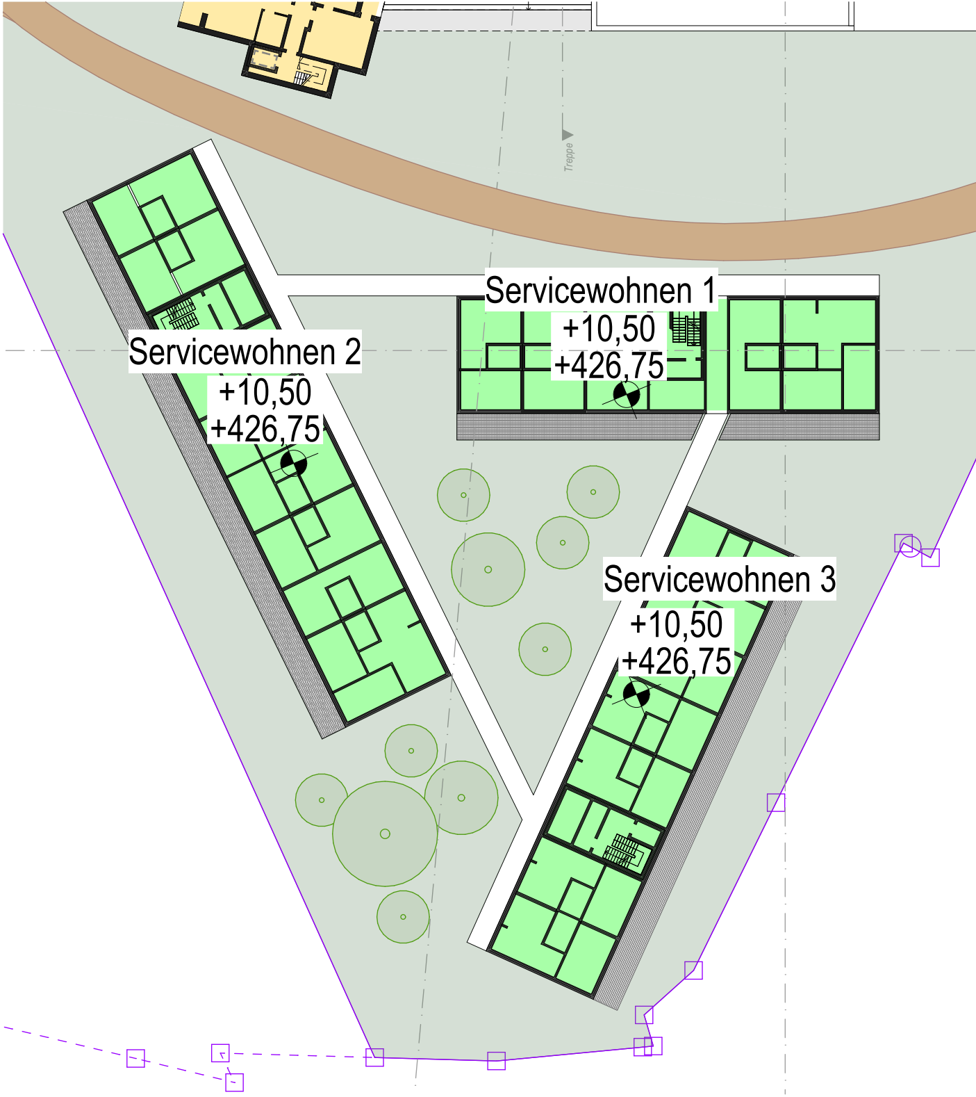
Servicewohnen Erdgeschoss
