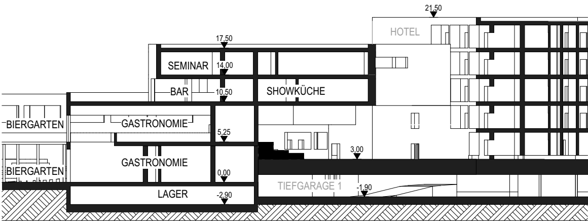
Schnitt Gastronomie
