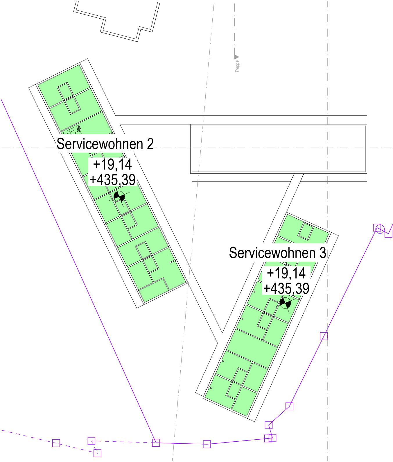
Servicewohnen 3. Obergeschoss
