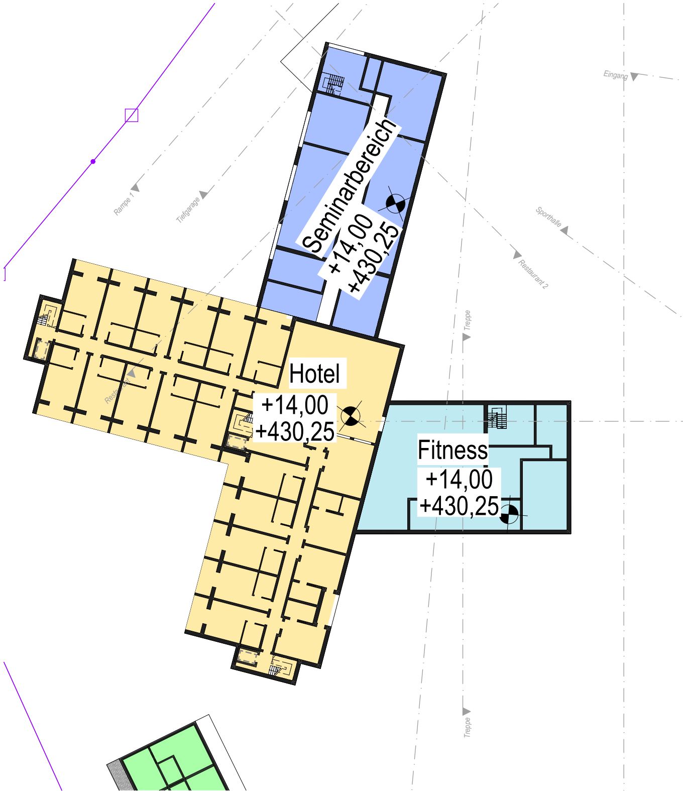
Hotel Obergeschoss 3
