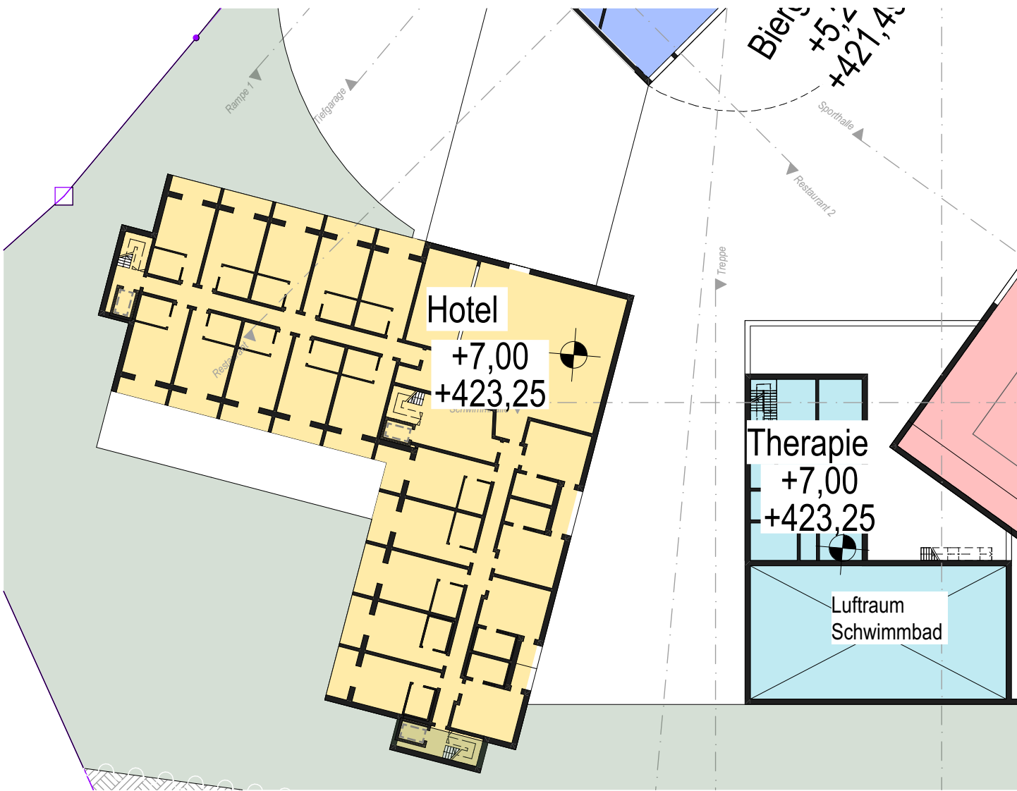
Hotel Obergeschoss 1
