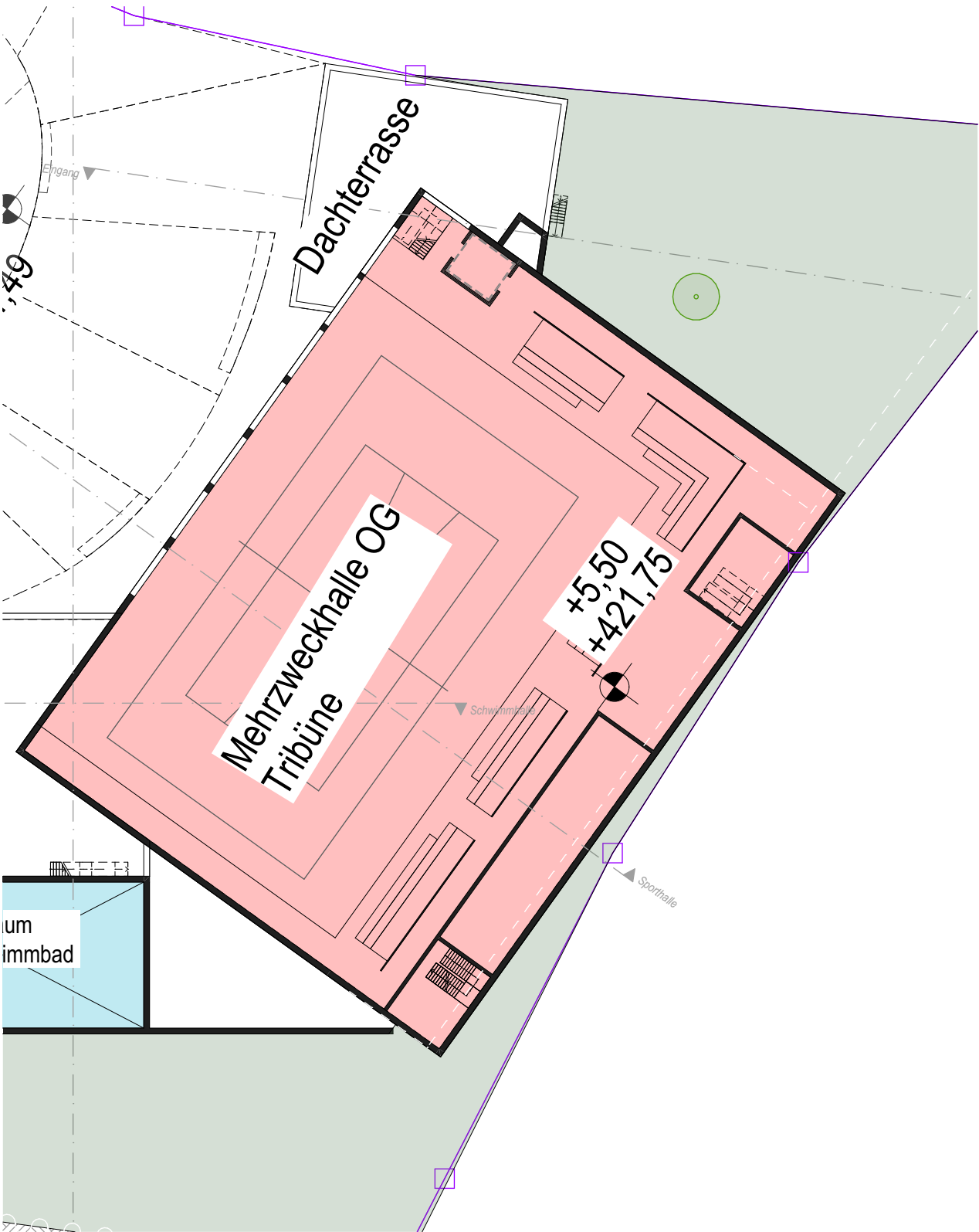
Sportbereich Obergeschoss
