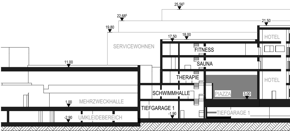
Schnitt Schwimmbad
