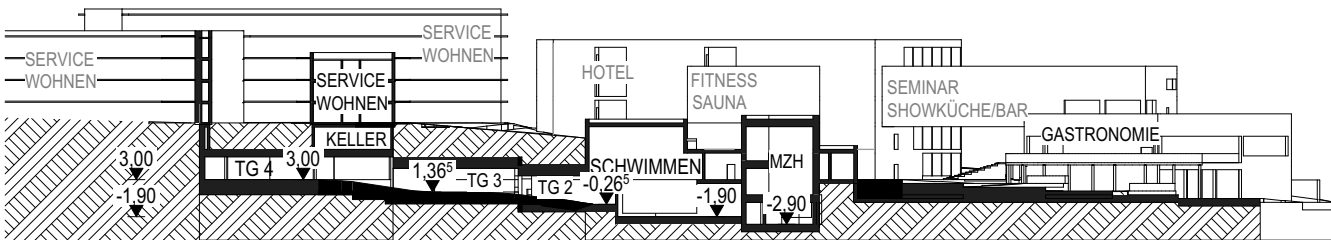
Schnitt Tiefgarage
