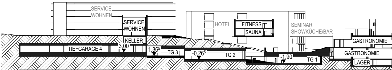
Schnitt Tiefgarage S2
