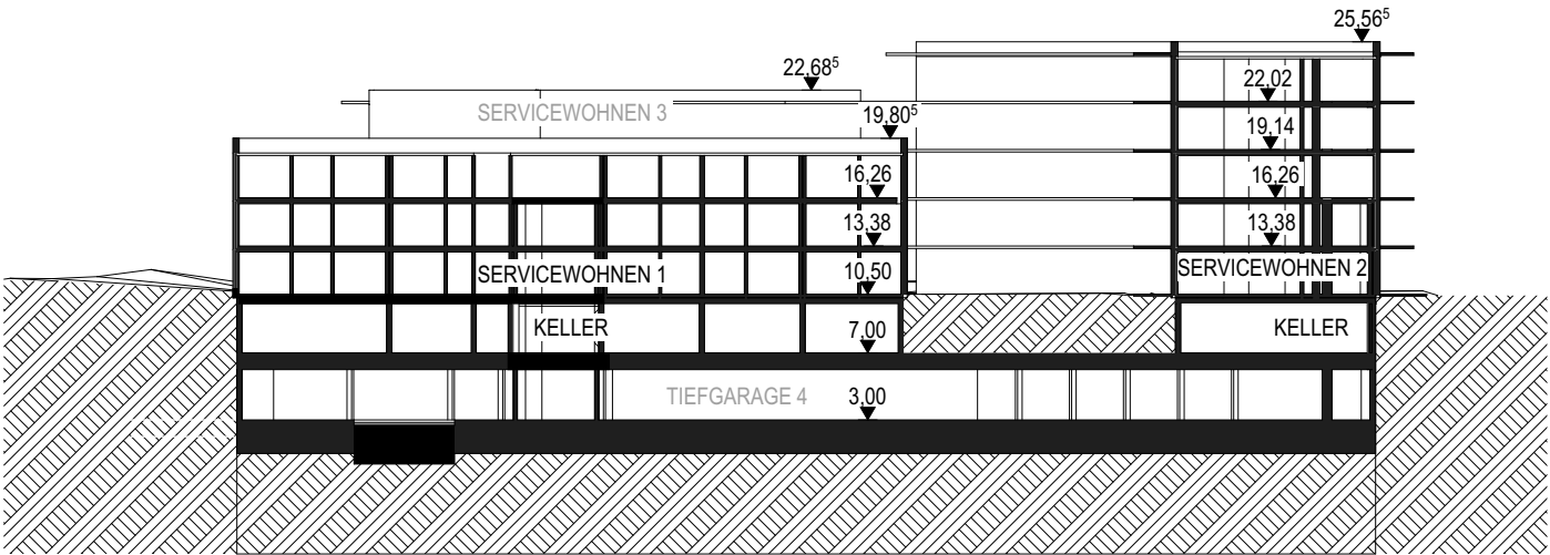
Schnitt Servicewohnen
