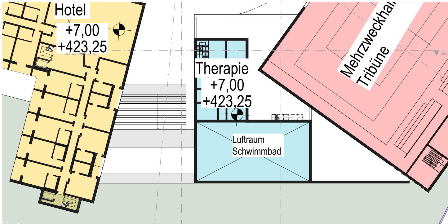
Therapie 1. Obergeschoss
