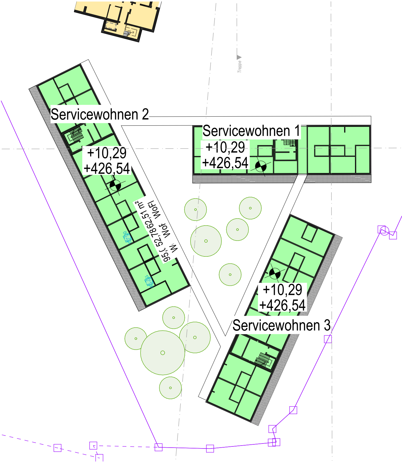
Servicewohnen 1. Obergeschoss
