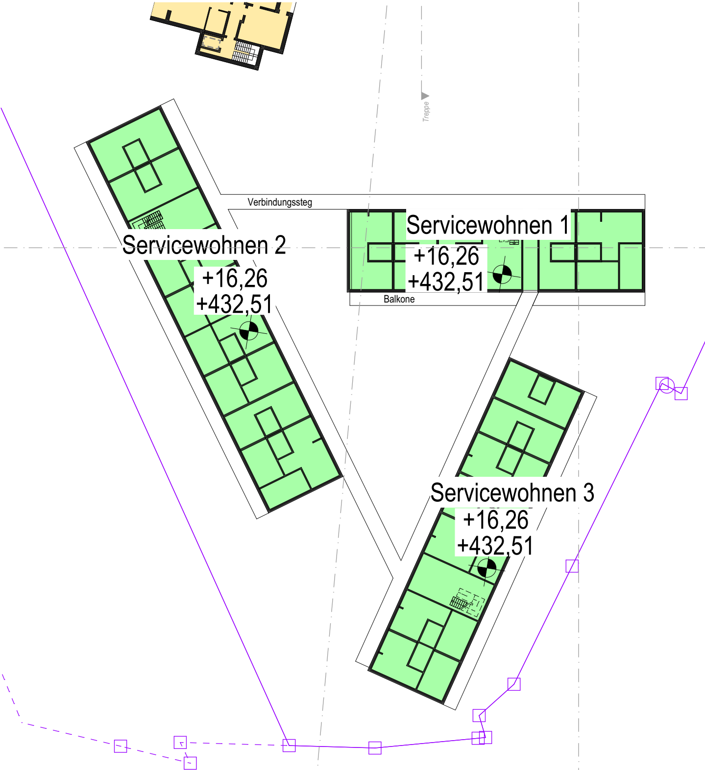
Servicewohnen 2. Obergeschoss
